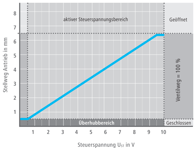
Beispielhaftes Funktionsdiagramm eines APV 40625-00
